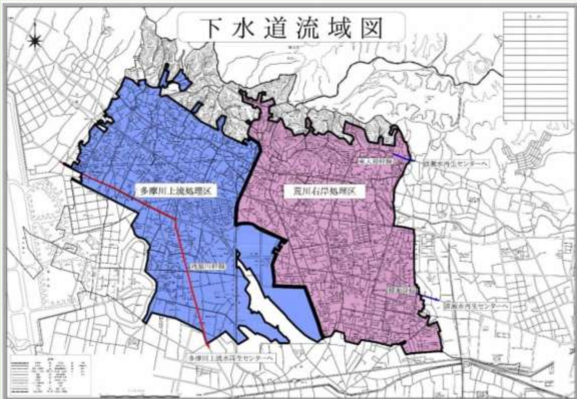
図 4-7 下水道流域図
