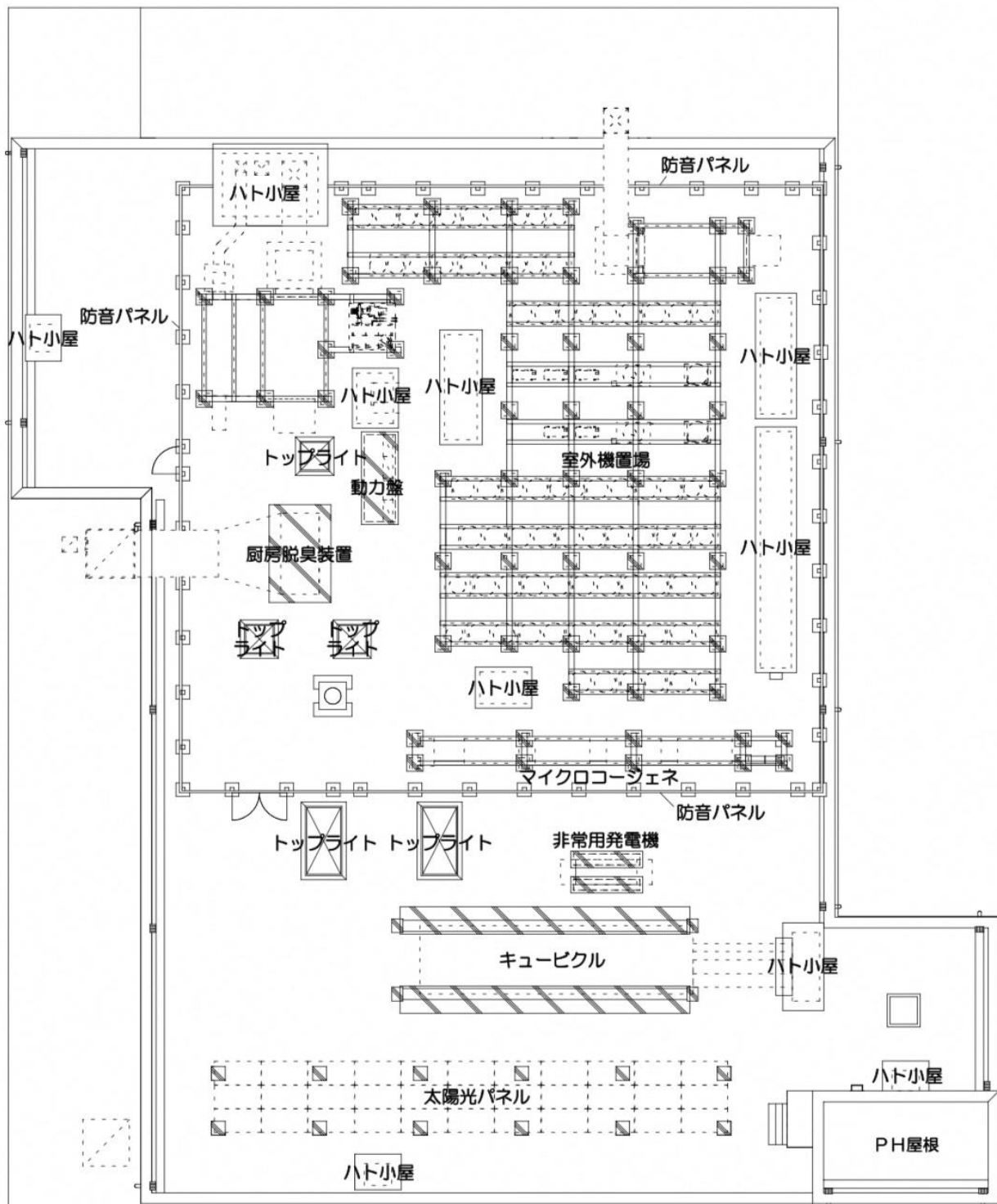
R 階平面図
